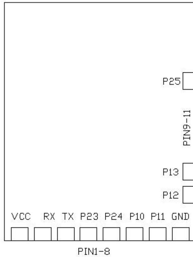
YH-007_V1.0 的引脚
