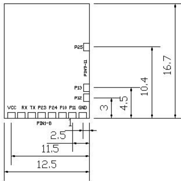
YH-007_V1.0 模块的外形尺寸
