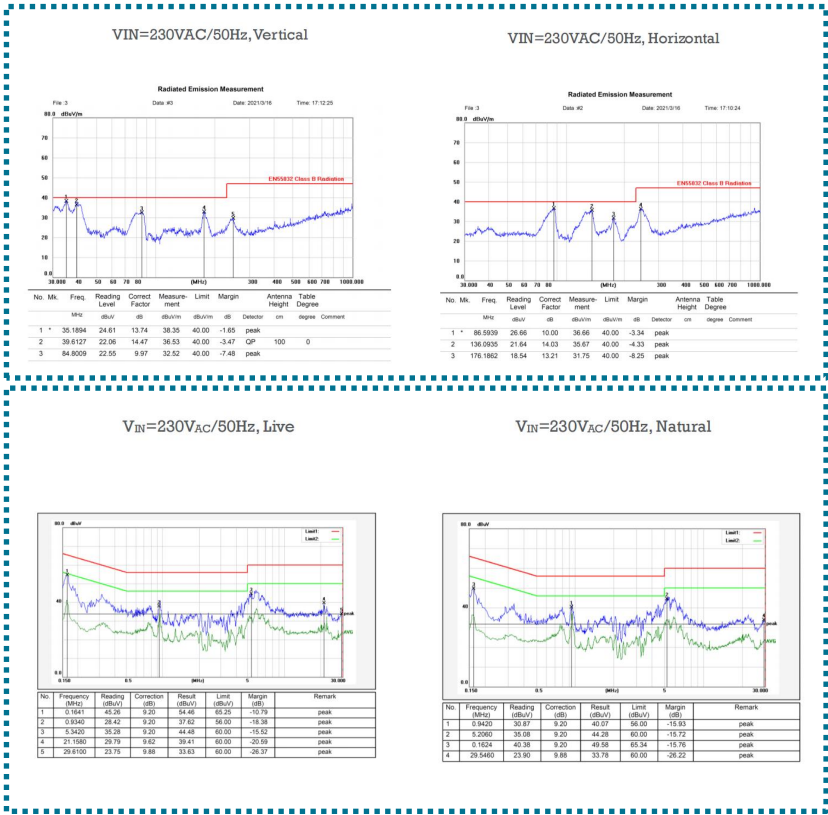
AC:230V 35W传导与辐射测试
